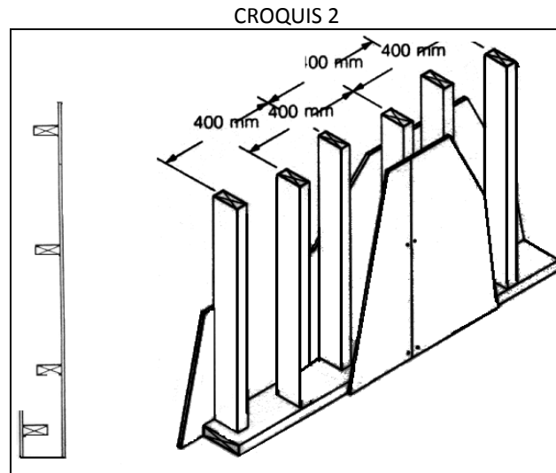
c) Murs de blocs de béton, 150 mm ( croquis 3 )
